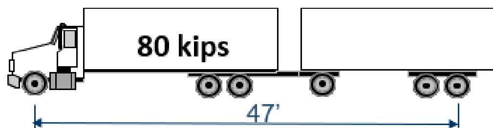
Type M3S3-40
